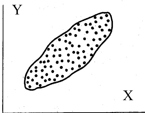
Рисунок 2 – Корреляционное поле, показывающее линейную зависимость числа подтягиваний (Y) от относительной силы мышц (X)
