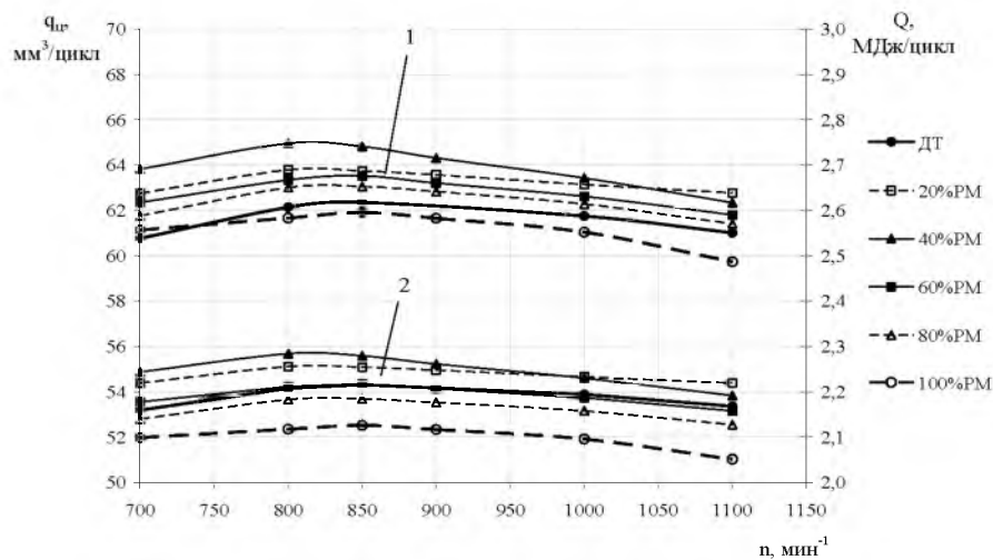
Рисунок 3. Скоростная характеристика топливного насоса: а – смесевые топлива с концентрацией рапсового масла до 20%; б – смесевые топлива с концентрацией рапсового масла до 100%; q_c – цикловая подача топлива (1); Q – вводимая с топливом теплота за цикл (2)
