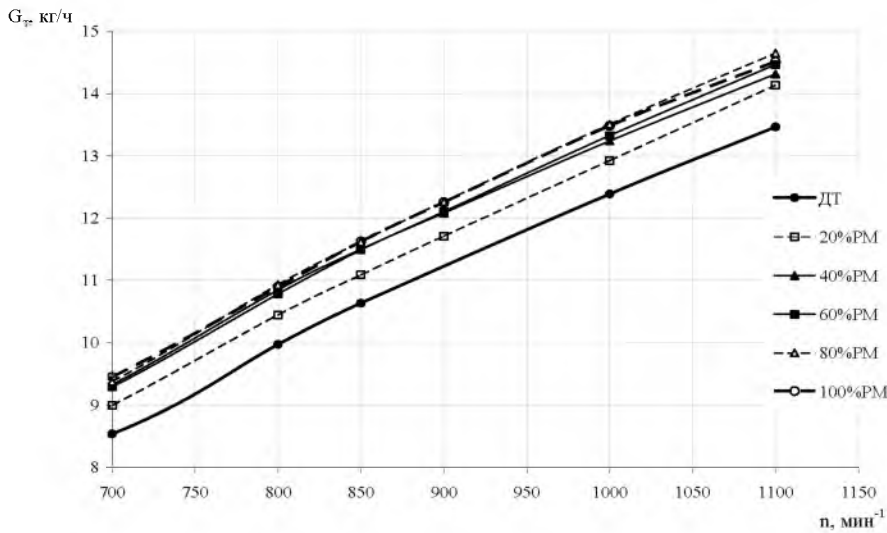
Рисунок 4. Часовой расход топлива:
