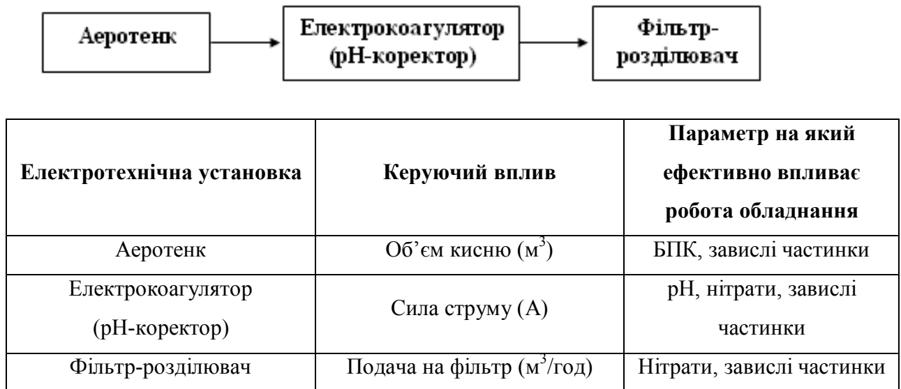
Рис. 3. Структура електротехнічного комплексу очистки стічних свиногокомплексу (укрупнено)
