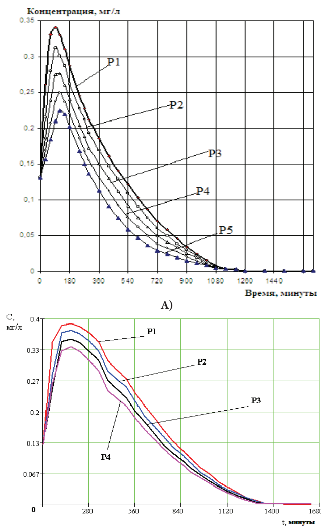
Рисунок 4. Динамика изменения концентрации осаждаемых веществ в контрольных пробах ёмкости при различных значениях давления: А – на выходе станции II-го подъёма; Б – в точке на расстоянии 7 километров от станции II-го подъёма (P1 – 0,06 МПа; P2 – 0,04 МПа; P3 – 0,02 МПа; P4 – 0 МПа (переходное состояние), P5 – -0,02 МПа (вакуумметрическое состояние))
