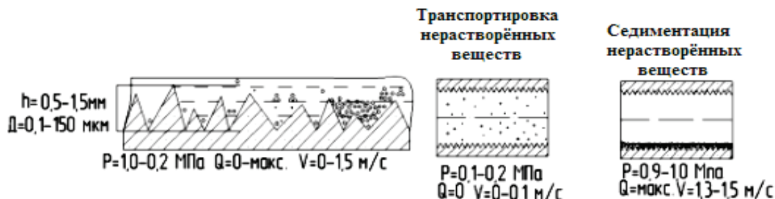
Рисунок 2. Графическое представление процесса накопления биологического загрязнителя воды в трубопроводе
