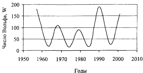
Рис. 3. Тренд солнечной активности за период 1958-2003 гг.
