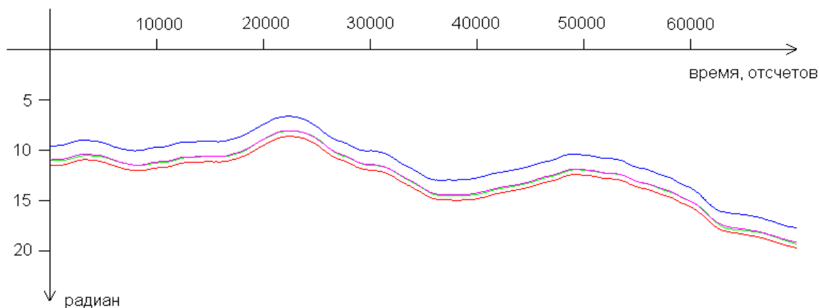
Рисунок 2. Фазы нижних мод, несомых целыми частотами, деленные на номер частоты (нормированные фазы). Звук «О», респондент Митянок. Частота дискретизации 44100 Гц. Базовая мода – красный цвет, вторая мода – фиолетовый, третья – зеленый, четвертая – синий. Образец N5.
