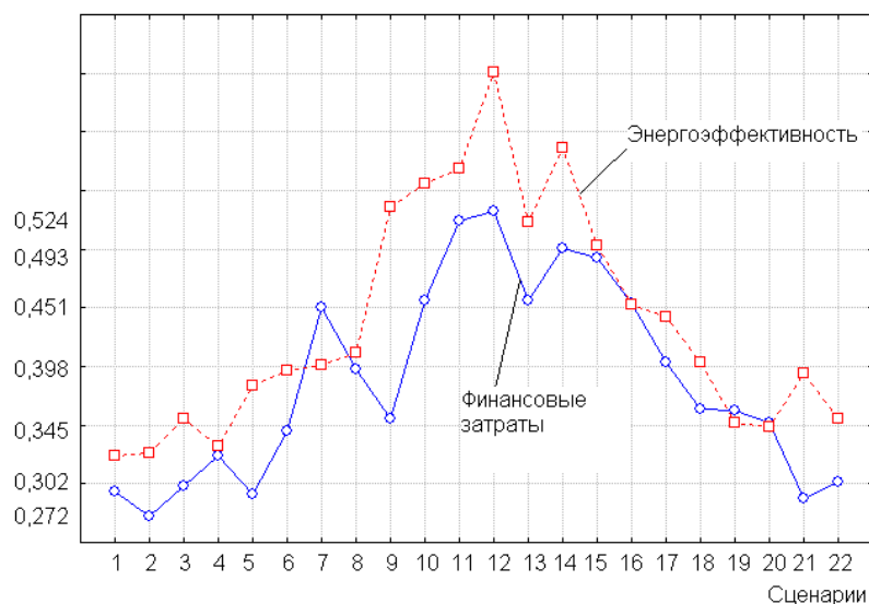
Рис. 2. Результаты сценарно-когнитивного моделирования комбинированных систем водоочистки
