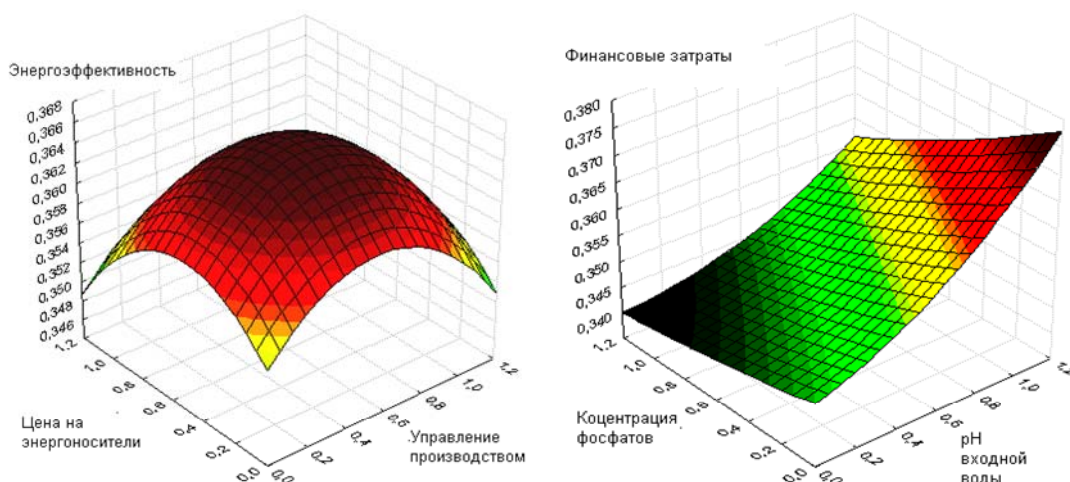
Рис. 5. Зависимости выходных концептов («Энергоэффективность» и «Финансовые затраты») от промежуточных и входных концептов (результаты работы оптимизированной нейросети)
