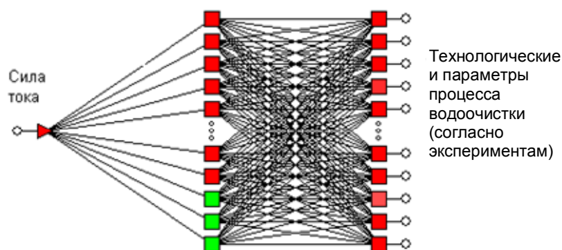
Рис. 6. Архитектура нейросетевой модели процессов водоочистки: учебная выборка – 2,42 %, контрольная выборка – 3,84 %, тестовая выборка – 3,75 %
