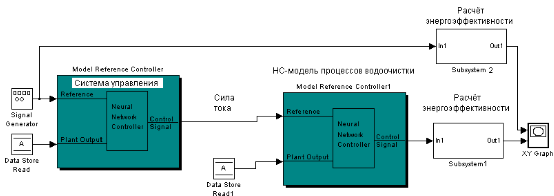
Рис. 7. Структура имитационного моделирования комбинированных систем водоочистки
