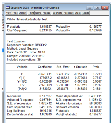
Рисунок 10 – Тест Уайта
