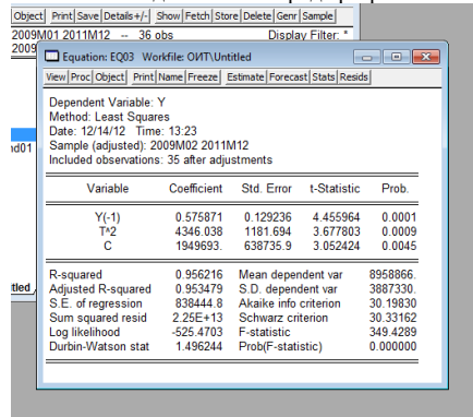
Рисунок 3 – Модель зависимости объемов реализации продукции от тренда и ряда приростов исходного ряда
