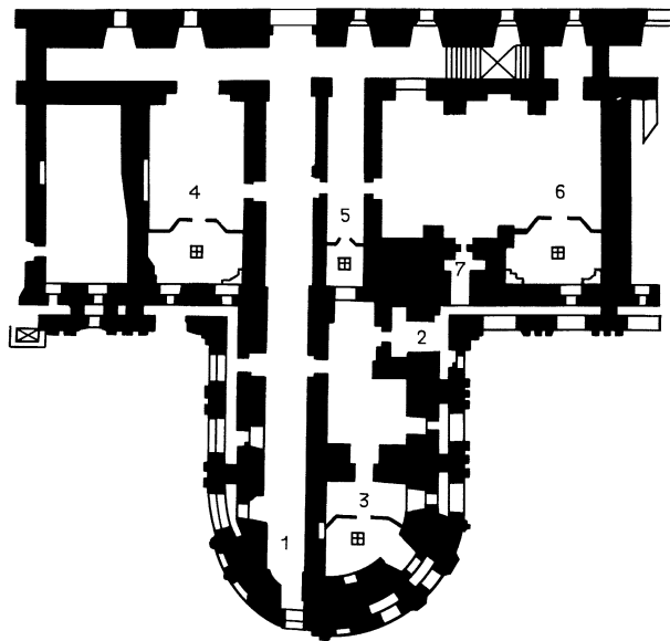
План храма Рождества Христова – «Вифлеемские церкви» (подклет) Конец XVIII – начало XIX в.
