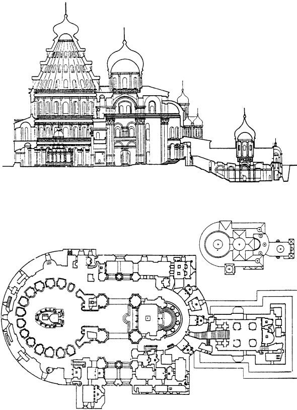
Ново-Иерусалимский монастырь. Воскресенский собор Разрез и планы сводов и первого этажа (обмеры из коллекции Музея архитектуры им. А.В. Щусева)
