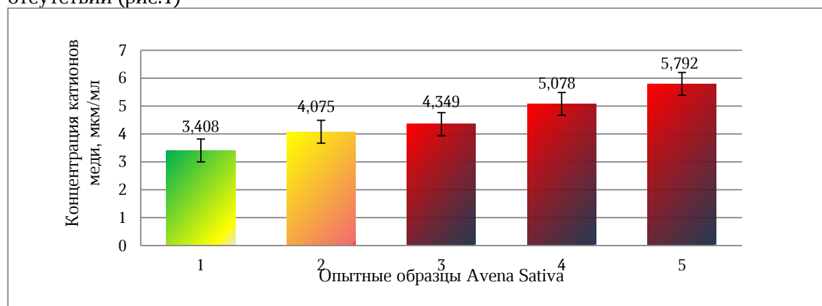
Рисунок 1. – Концентрации ионов меди в клеточном соке овса посевного
